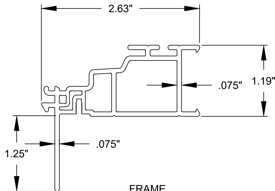
FRAME (VINYL)
